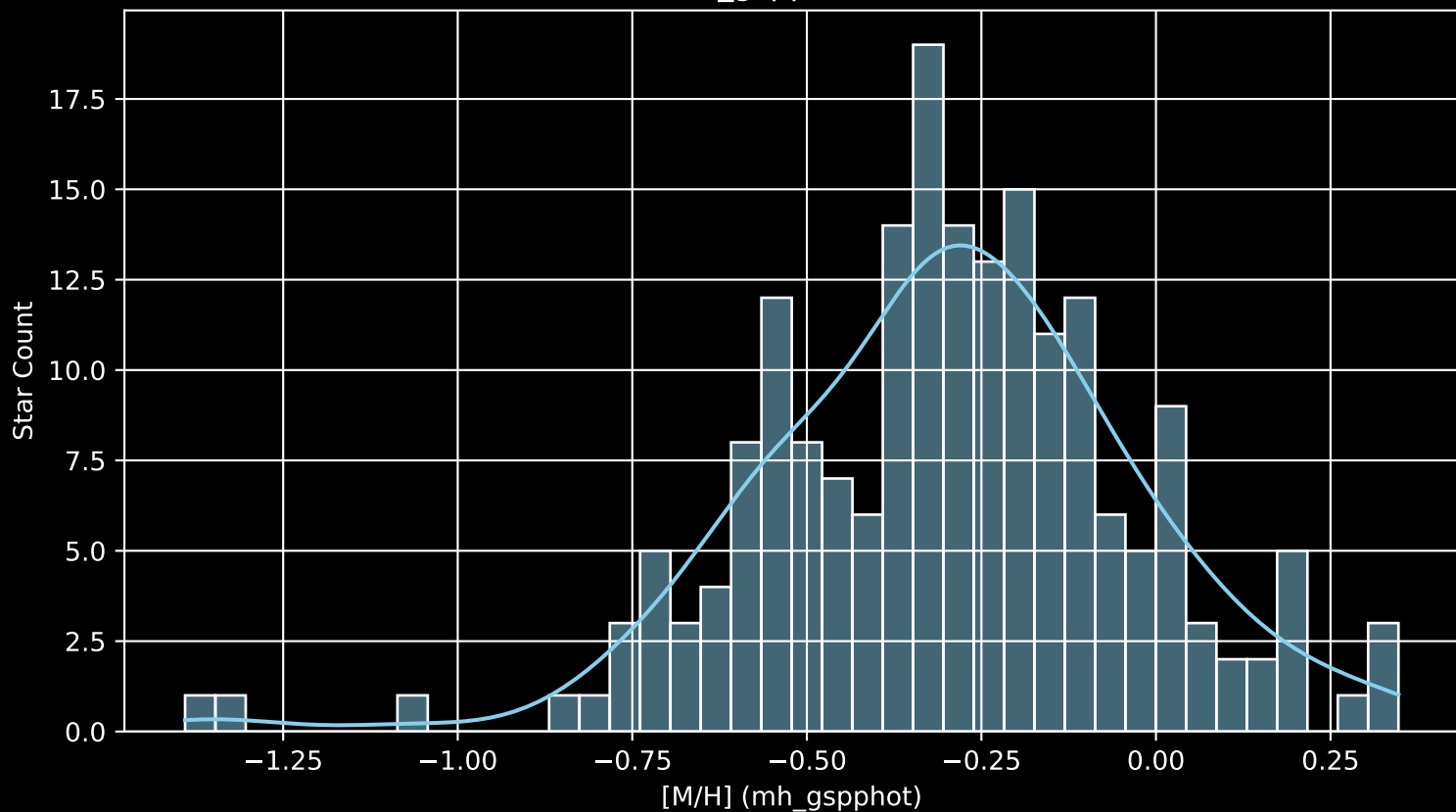
GALAH DR4 Field: [338] [M/H] (mh_gspphot) (n= 195)
