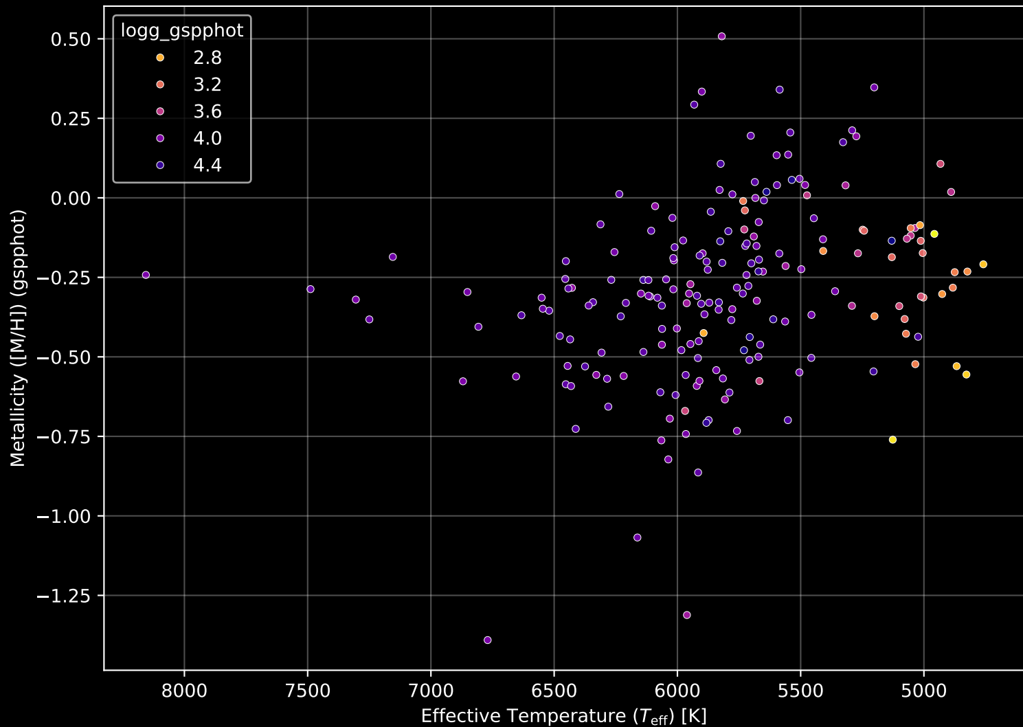
GALAH DR4 Field: [338] Stellar Population Parameters (n= 196)
