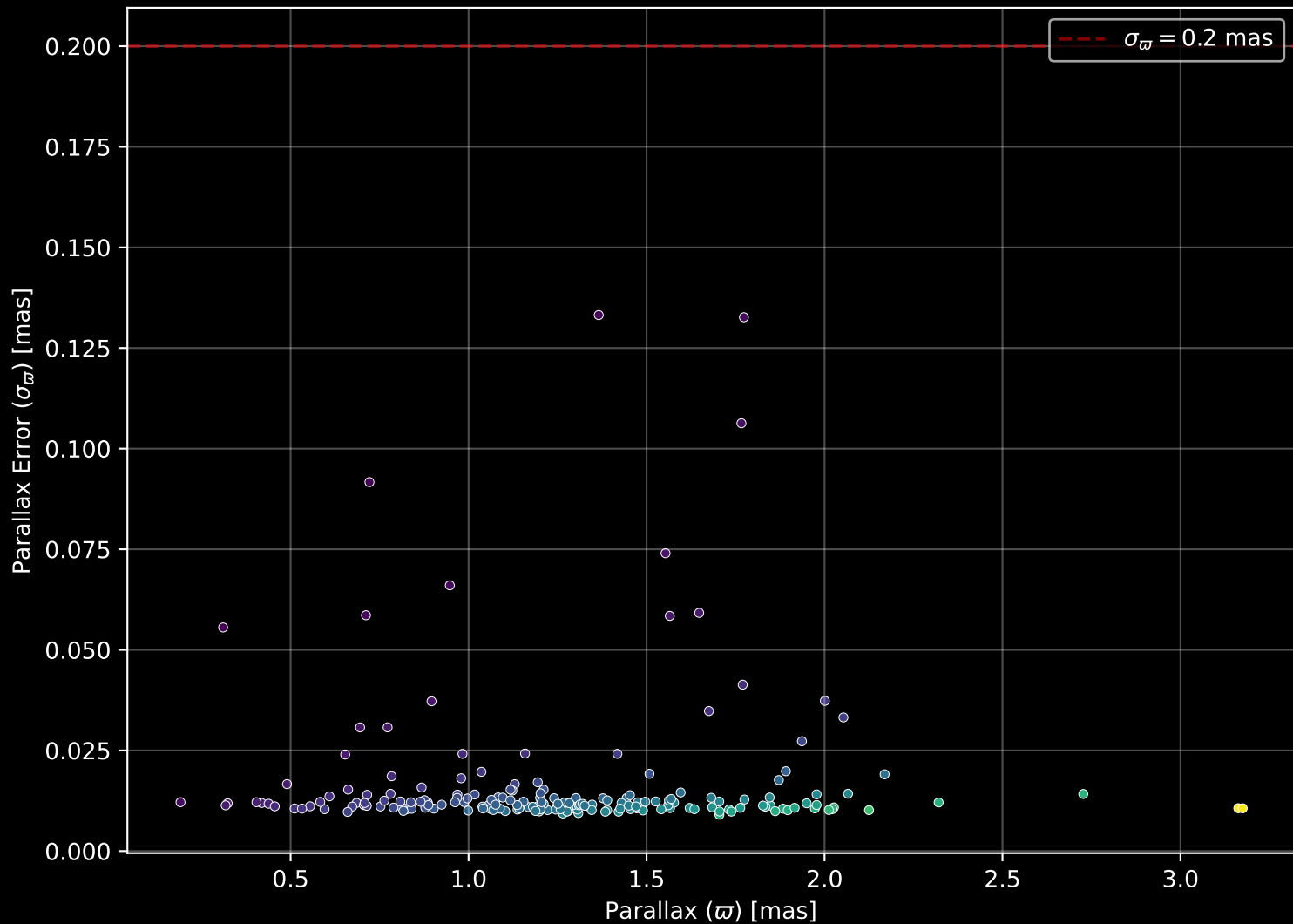
GALAH DR4 Field: [338] Parallax Quality (n= 196)
