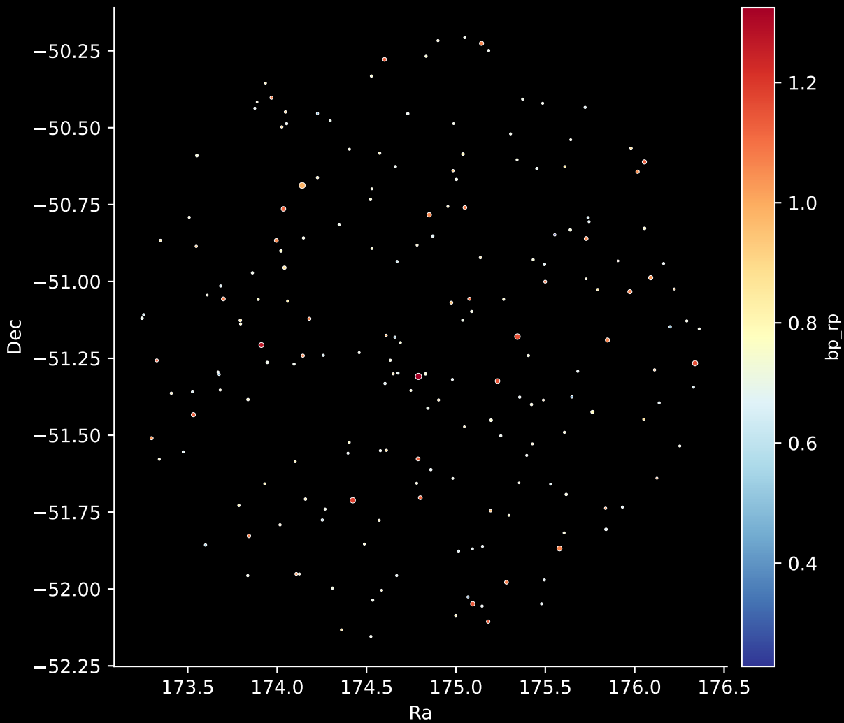
GALAH DR4 Field: [338] Stars: 196
